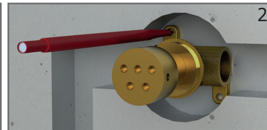
2 NIVELAR EL CUERPO (NIVEL NO INCLUIDO) LEVEL THE BODY (LEVEL NOT INCLUDED)
