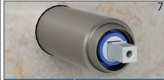
7 REALIZAR UNA PERFORACIÓN EN LA LOSA DONDE ENTRE FACILMENTE EL CUERPO DE LA GRIFERÍA DRILL A HOLE IN THE SLAB WHERE THE BODY OF THE FAUCET CAN EASILY ENTER.
