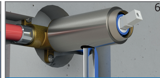
6 COMPROBAR EL CORRECTO FUNCIONAMIENTO ANTES DE CERRAR CHECK FOR PROPER OPERATION BEFORE CLOSING
