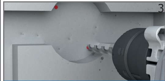
3 MARCAR EN LA PARED LOS HUECOS PARA REALIZAR LOS ORIFICIOS Y TALADRAR MARK ON THE WALL THE HOLES TO DRILL AND DRILL THE HOLES
