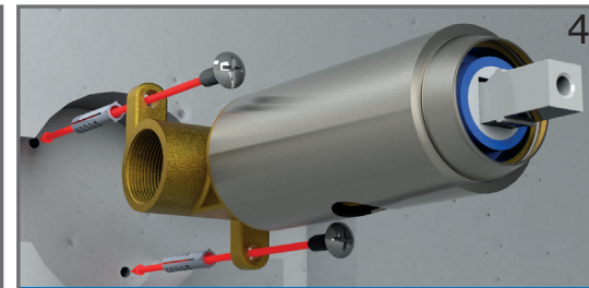
4 COLOCAR LOS TACOS EN LOS ORIFICIOS Y EL CUERPO ENCIMA CON TORNILLOS PARA FIJARLO A LA PARED PLACE THE DOWELS IN THE HOLES AND THE BODY ON TOP WITH SCREWS TO FIX IT TO THE WALL
