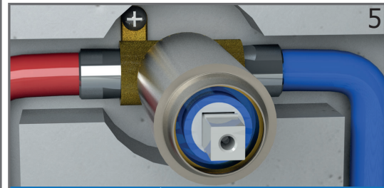
5 INSTALAR LAS TUBERÍAS CON SUS RACORES Y CINTA DE TEFLÓN PARA EVITAR FUGAS INSTALL THE PIPES WITH THEIR FITTINGS AND TEFLON TAPE TO PREVENT LEAKS
